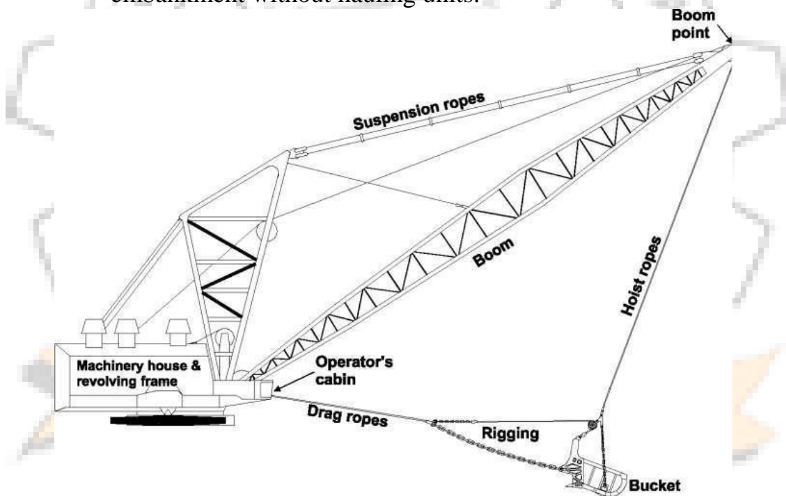
Fig. Dragline
