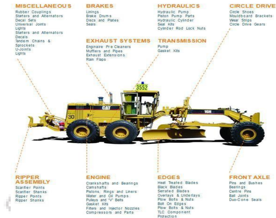
Fig. Grader
